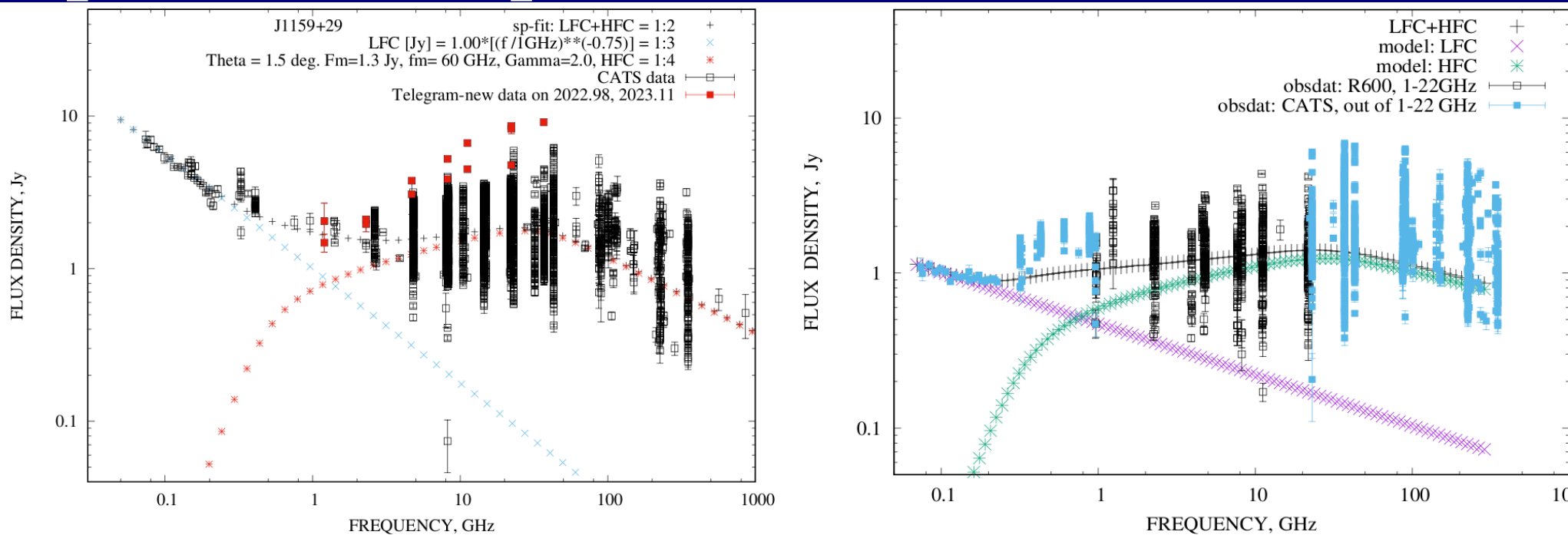
Рис. 2. Модельные исследования физических параметров в протонных струях, условий ускорения протонов для генерации нейтрино + РСДБ-структур у СМЧД.
